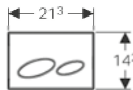
Geberit Kappa20 W 21.3 / D 1.5 / H 14.2cm
