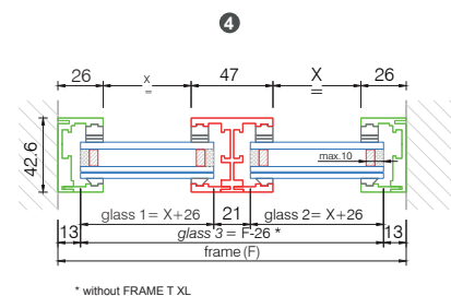
Horizontal section Frame XL/Frame T XL
