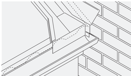
Fig. 28 – Secret gutter
