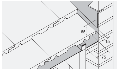
Fig. 29 – Secret gutter
