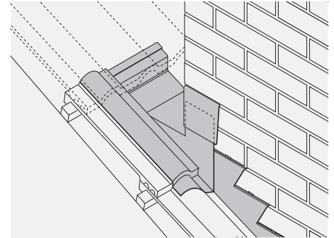
Fig. 31 – Back gutter
