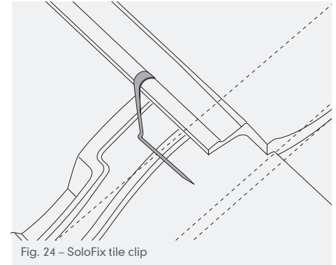
Fig. 24 – SoloFix tile clip
