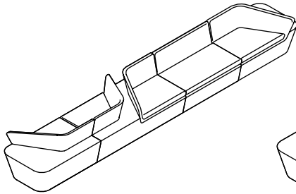
5 W4720 D760 H725 mm
