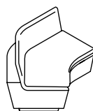
MS04 Angle 45 W1252/1040 D760 H725 mm
