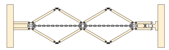
Duplo horizontal section
